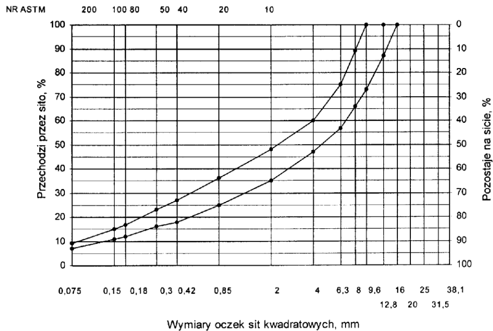
Rys. 6. Krzywe graniczne uziarnienia mieszanki mineralnej BA od 0 do 16 mm do warstwy ścieralnej nawierzchni drogi o obciążeniu ruchem od KR3 do
