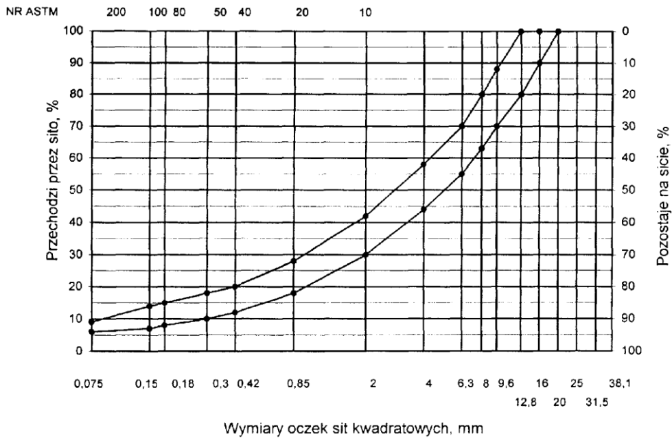
Rys. 6. Krzywe graniczne uziarnienia mieszanki mineralnej BA od 0 do 16 mm do warstwy ścieralnej nawierzchni drogi o obciążeniu ruchem od KR3 do
